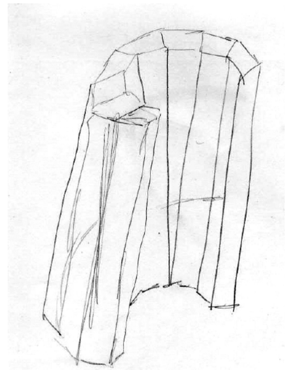
Skizze, Möglichkeit der Verleimung von Eichenbohlen
